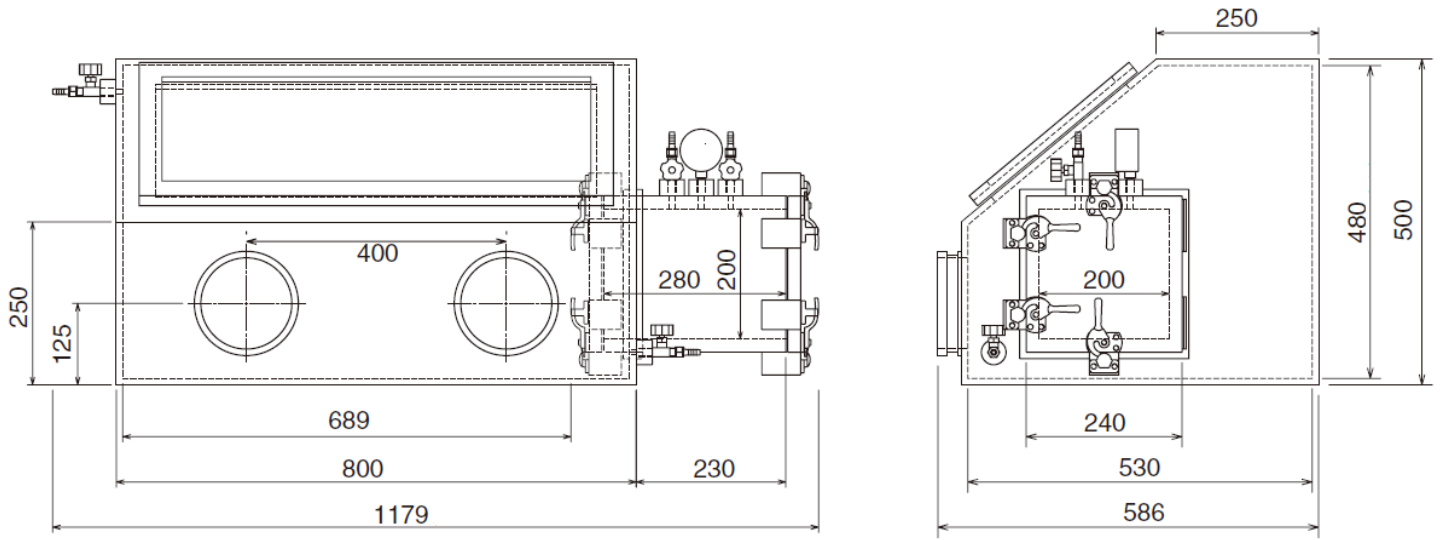
Чертеж DX-2 (размеры указаны в мм)
